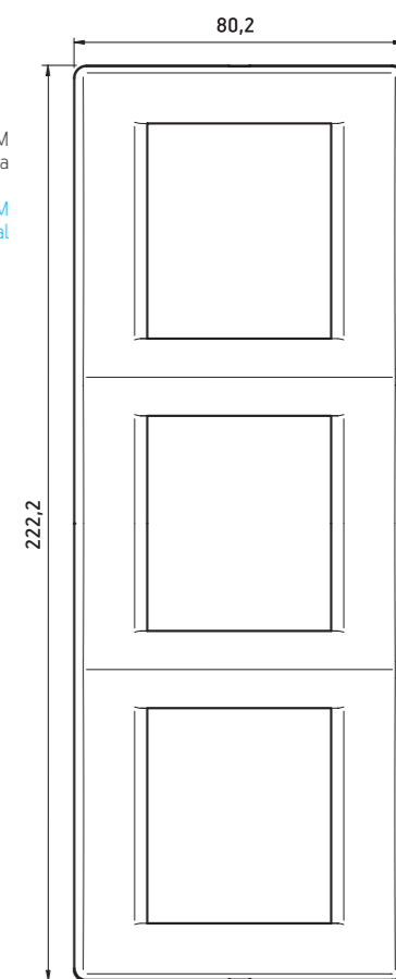
Maska višestruka 3x2M vertikalna
